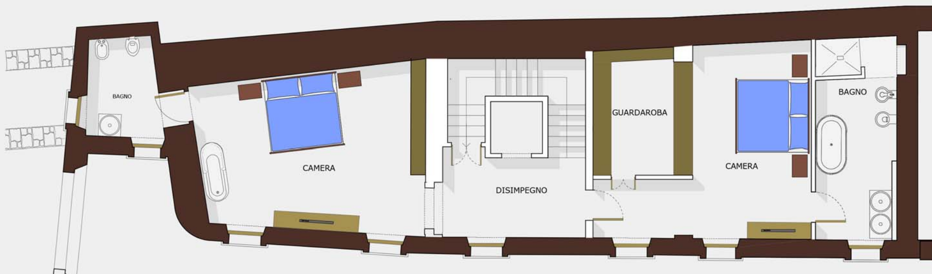
PIANTA PIANO PRIMO
